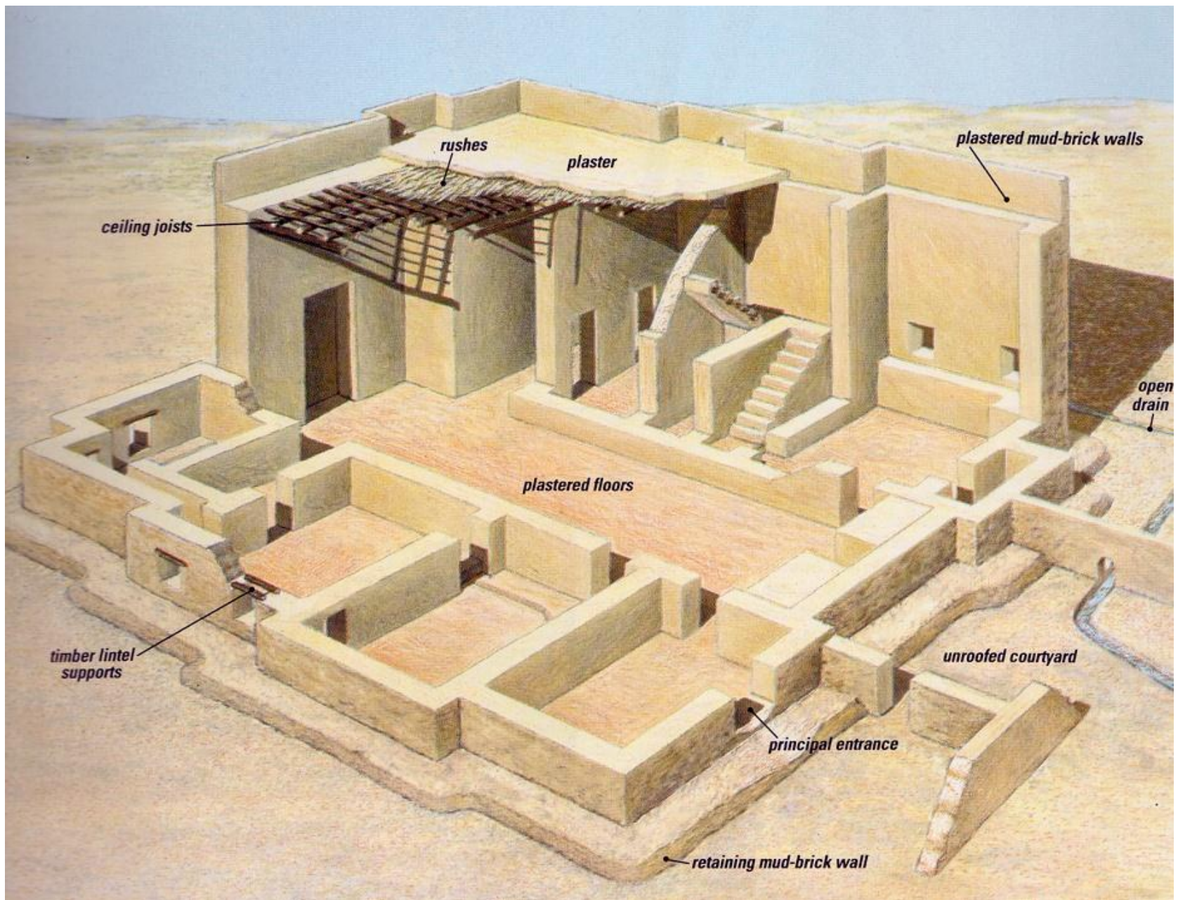
Arquitectura Tell Madhur, proposición de restitución (M. Roaf, 1982)
