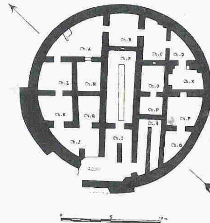
Plan et proposition de restitution du volume ancien de la Maison Ronde de Tepe Gawra ; au rez-de-chaussée la fonction réserve prédomine ; alors qu'à l'étage sont concentrées les fonctions de réception et de séjour (début 4e millénaire).
