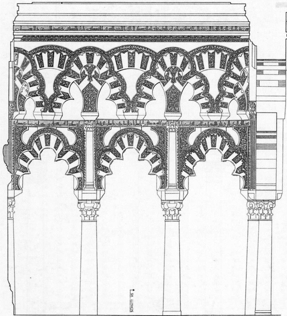
Fig. 7.- Córdoba, Gran mezquita, sala de oraciones, sistema de arcos entrecruzados VSS (situación: v. fig. 4; Ew 1968, boja VSS 1). 1: 50.
