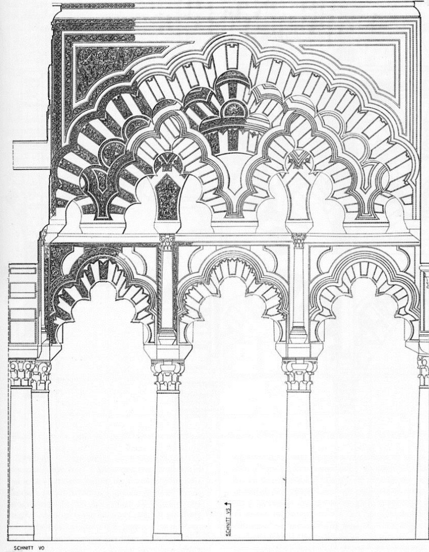
Fig. 8.- Córdoba, Gran mezquita, sala de oraciones, sistema de arcos entrecruzados VSN (situación: v. fig. 4; Ew 1968, boja VSN 1). 1: 50.
