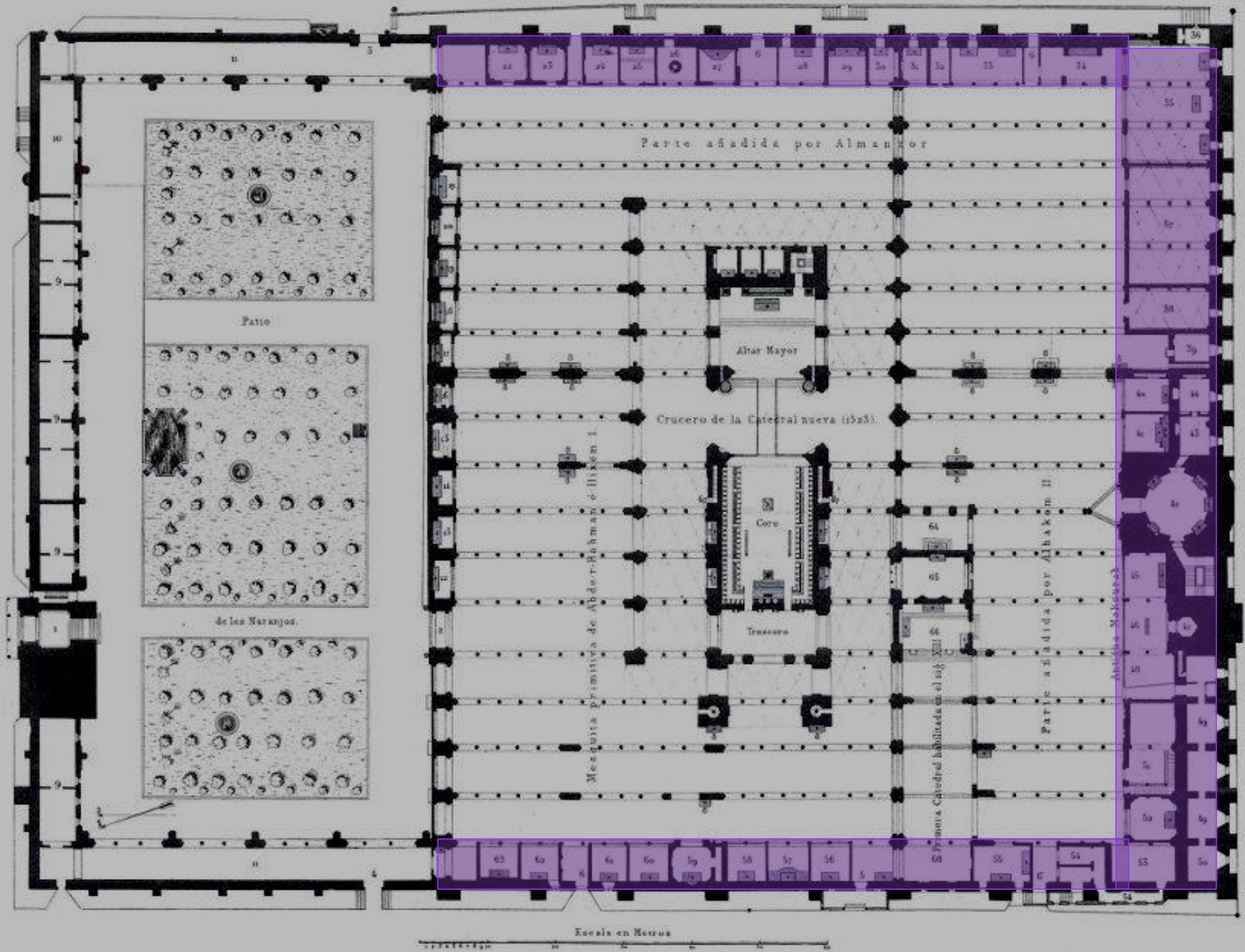
MEZQUITA Y CATEDRAL DE CÓRDOBA (PLANTA GENERAL).
